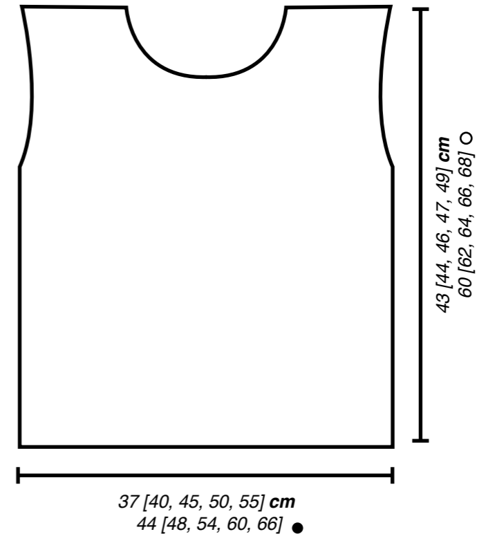
VORDER UND RÜCKTEIL
